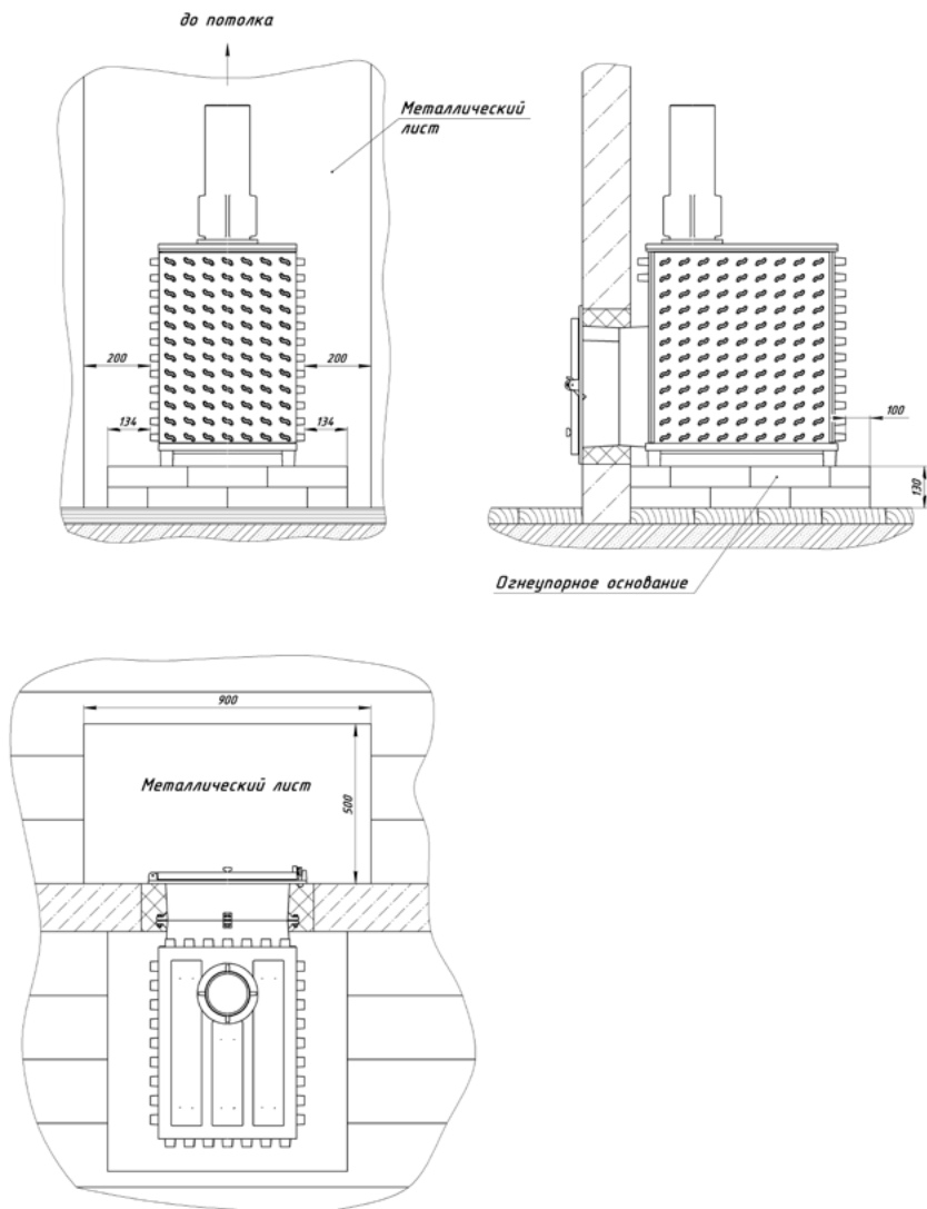
Рис.3 – Монтаж печи
