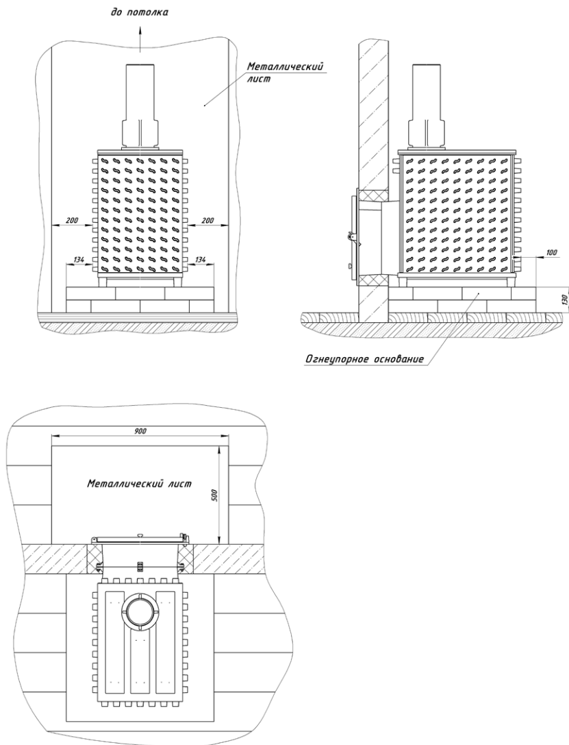
Рис.3 – Монтаж печи
